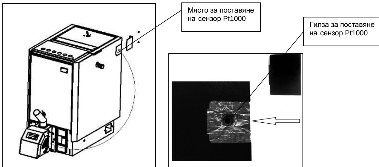
Фигура 14. Монтаж на сензора за температура на водата
