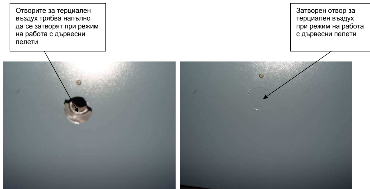
Фигура 8. Отвори за терциален (третичен) въздух, разположени на страничните капаци на котли серия Bisolid Saver W и Bisolid Saver C
